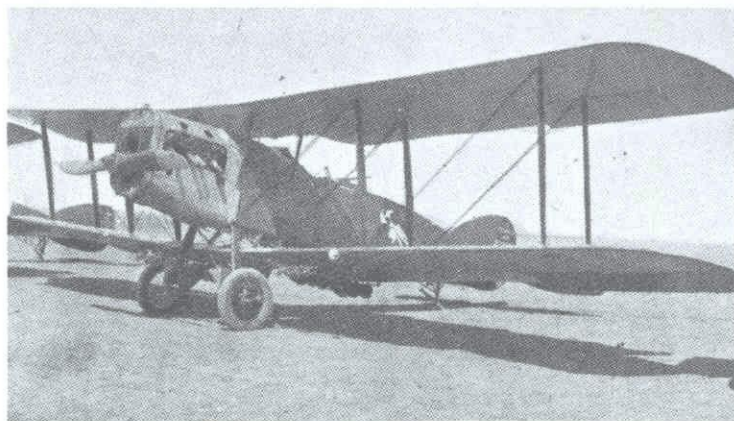
Bristol F2B , con motor Hispano-Suiza 8Fb de 300 CV.
